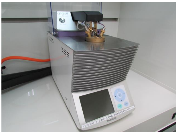
【タグ密閉式自動引火点試験器】
