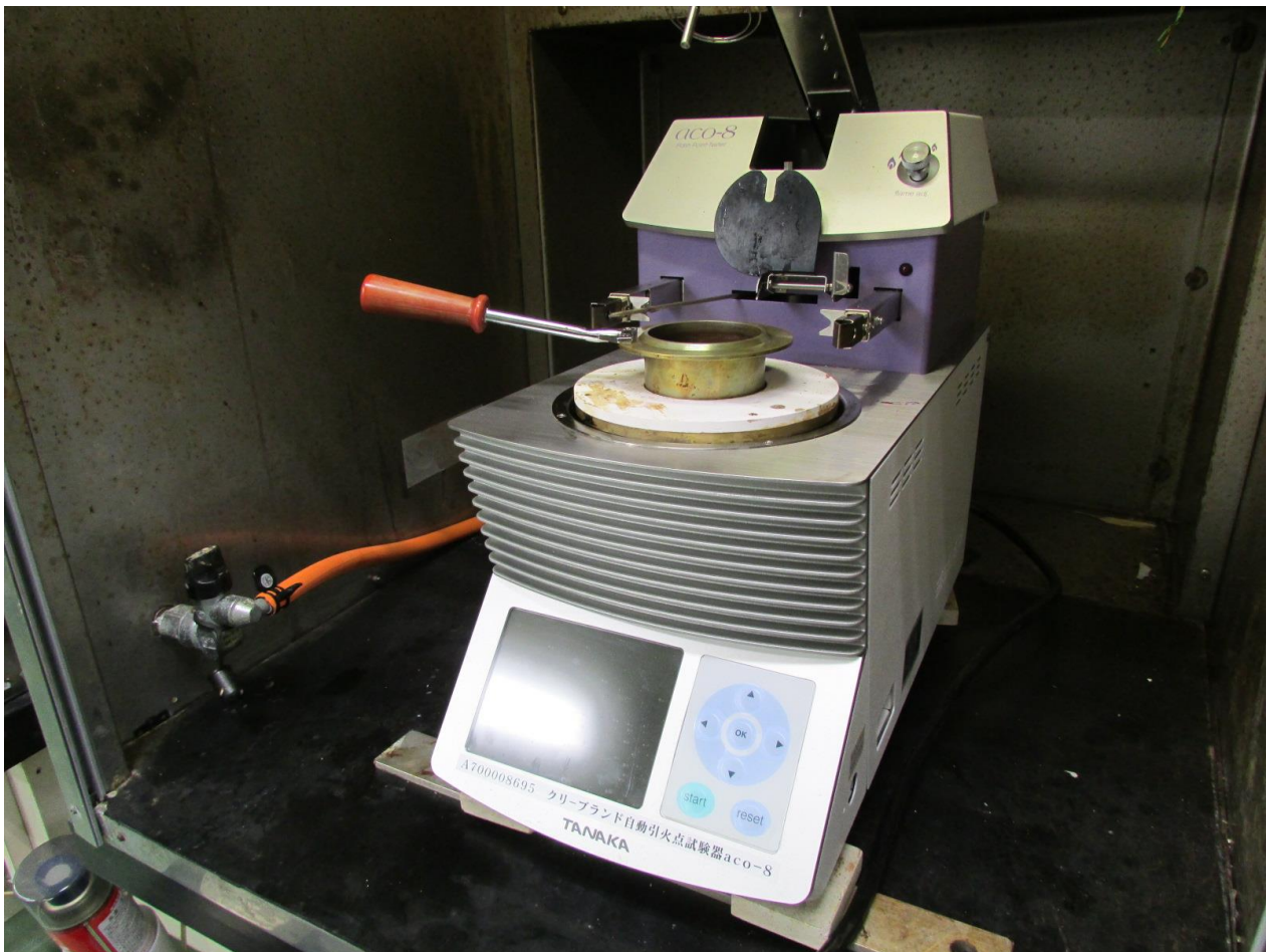
【クリーブランド開放式自動引火点試験器】
